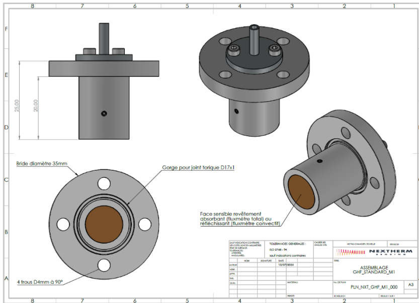
Fig.3 Fluxmètre GHF en interface mécanique à bride 4 trous à 90° (référence M1). La répartition des trous diffère de celle du capteur de gamme CHF (refroidi, 3 trous à 120°) pour éviter intersion et endommagement.
