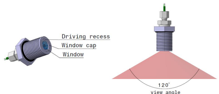
Fig.6 Fluxmètre radiatif : spectre de transmission à prendre en considération et aménagement du capteur
